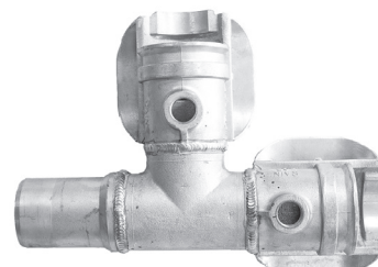
3" End Tee Aluminum RainTite™ Custom PN# 1012522
